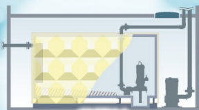
釜場付 パネルタンクユニット
